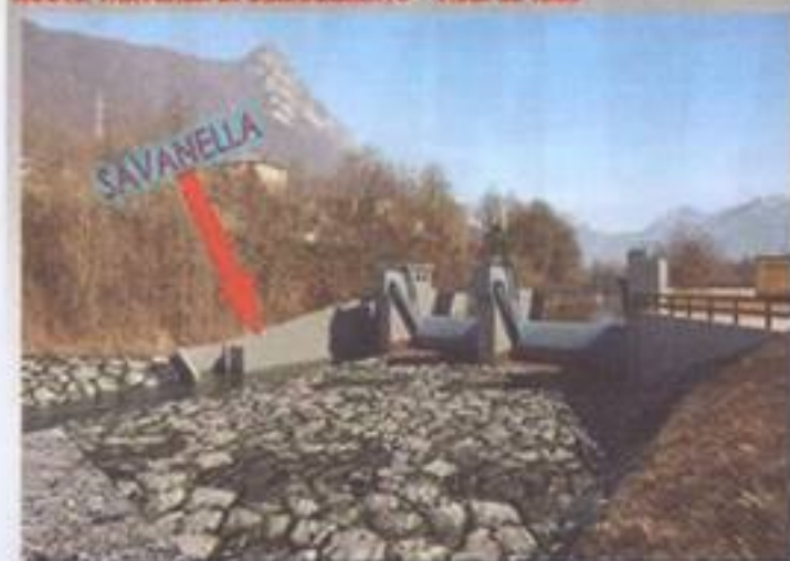
NUOVA TRAVERSA DI SBARRAMENTO - Vista da valle
