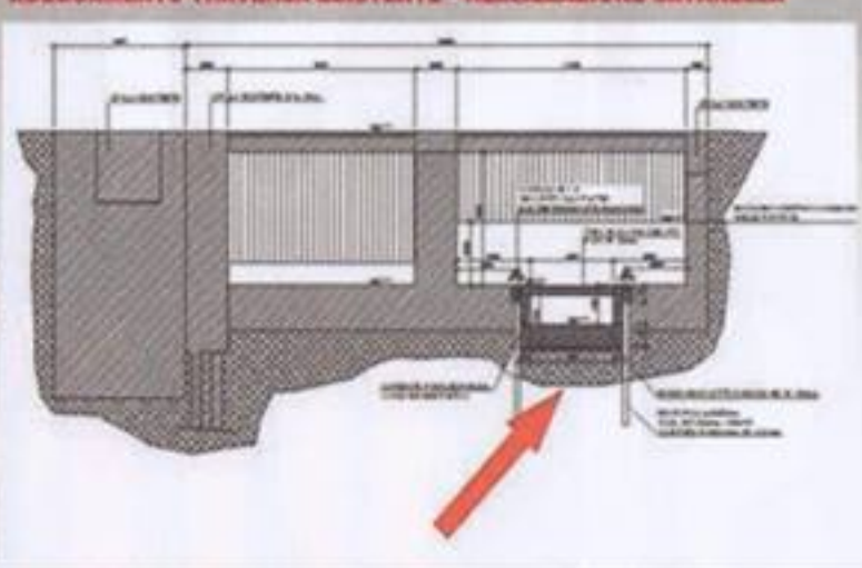
ADEGUAMENTO TRAVERSA ESISTENTE - REALIZZAZIONE SAVANELLA
