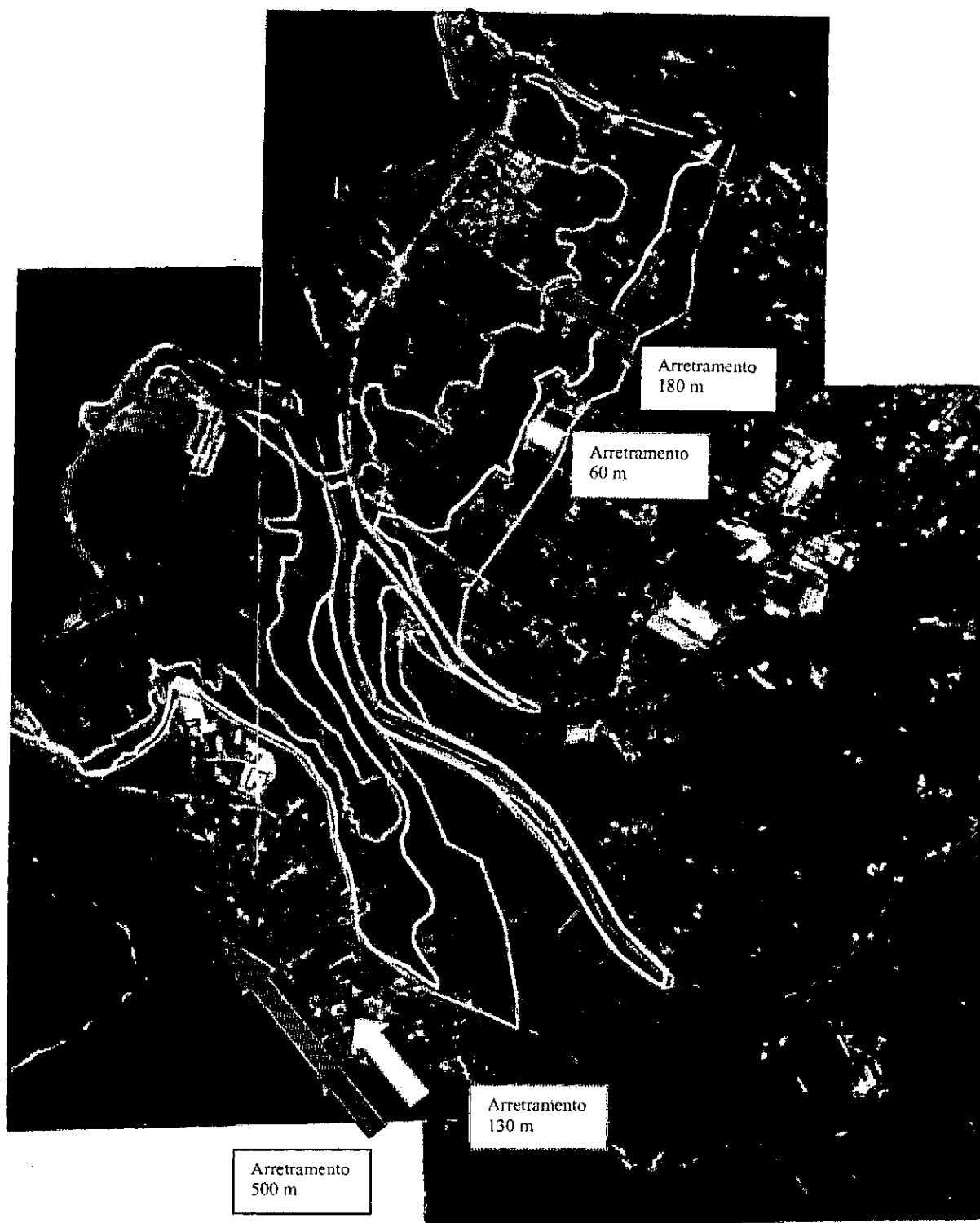
Figura 13: perimetrazione aree interessate da esondazione - piena T_r=1000 anni - idrogramma con singolo colmo. In azzurro stato di fatto ( H_{\text{lago}}=370,67 ), livello iniziale del lago a quota 365,20 m slm. In giallo ( H_{\text{lago}}=370,12 m slm), livello iniziale del lago a quota 365,20 m slm. In verde ( H_{\text{lago}}=368,97 m slm) livello iniziale del lago a quota 364,75 m slm.
